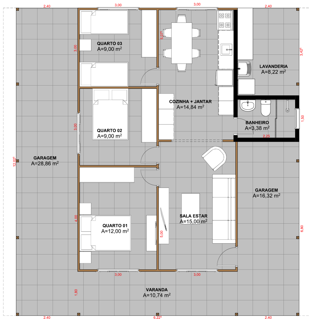
Modelo 78 • Casa Modelo Chácara Praia (6x10 tipo 02) • Marca atualizada para Construtora Silva.
