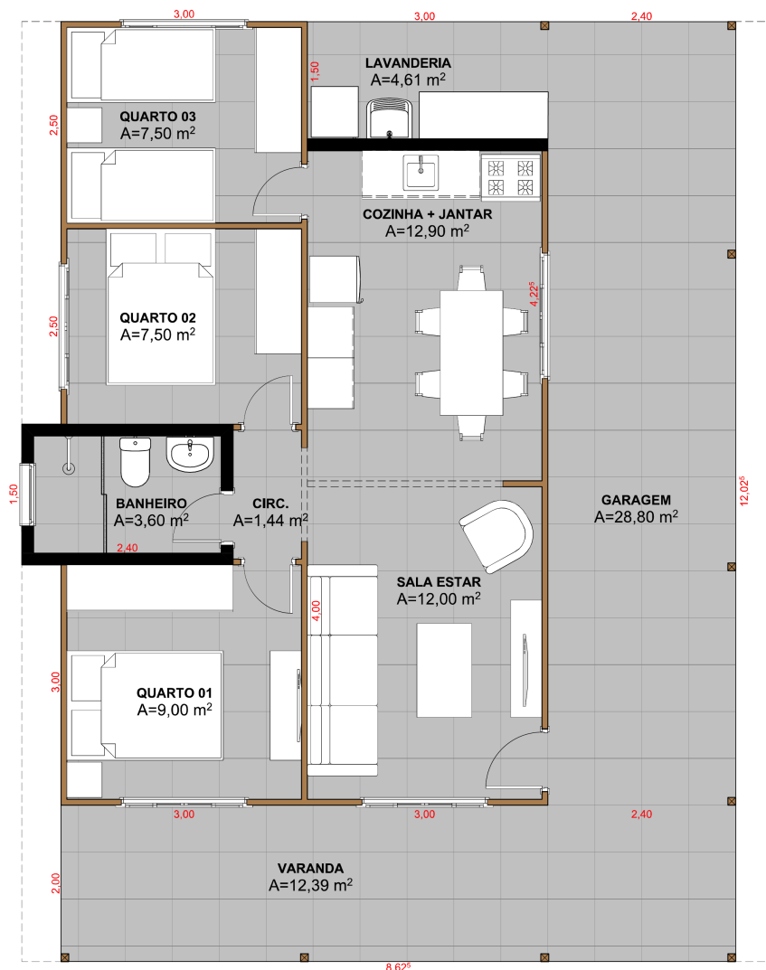
Modelo 13 • Casa Modelo Frente Dupla (6x8) • Marca atualizada para Construtora Silva.
