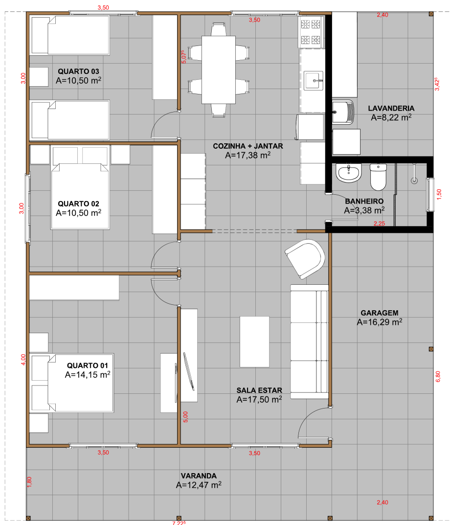
Modelo 35 • Casa Modelo Convencional (7x10) • Marca atualizada para Construtora Silva.
