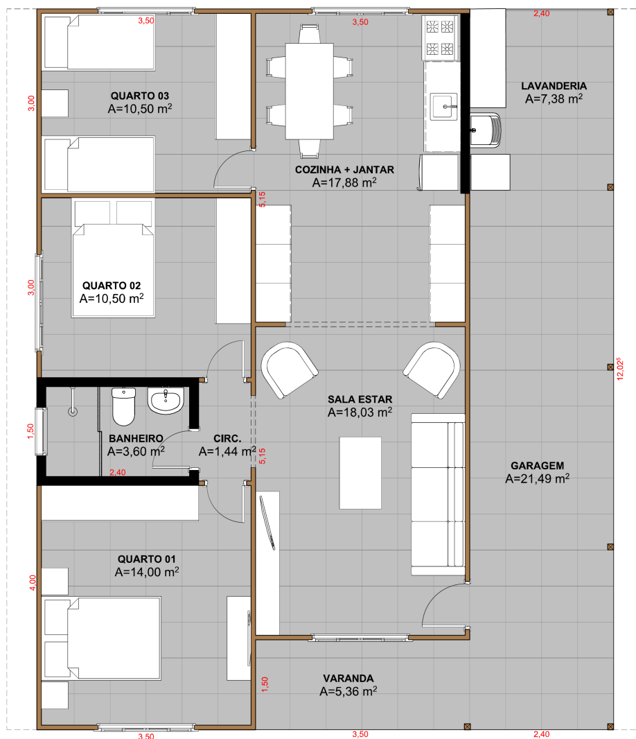
Modelo 24 • Casa Modelo Construtora Silva (7x10) • Marca atualizada para Construtora Silva.
