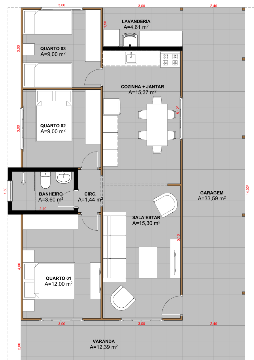
Modelo 15 • Casa Modelo Frente Dupla (6x10) • Marca atualizada para Construtora Silva.
