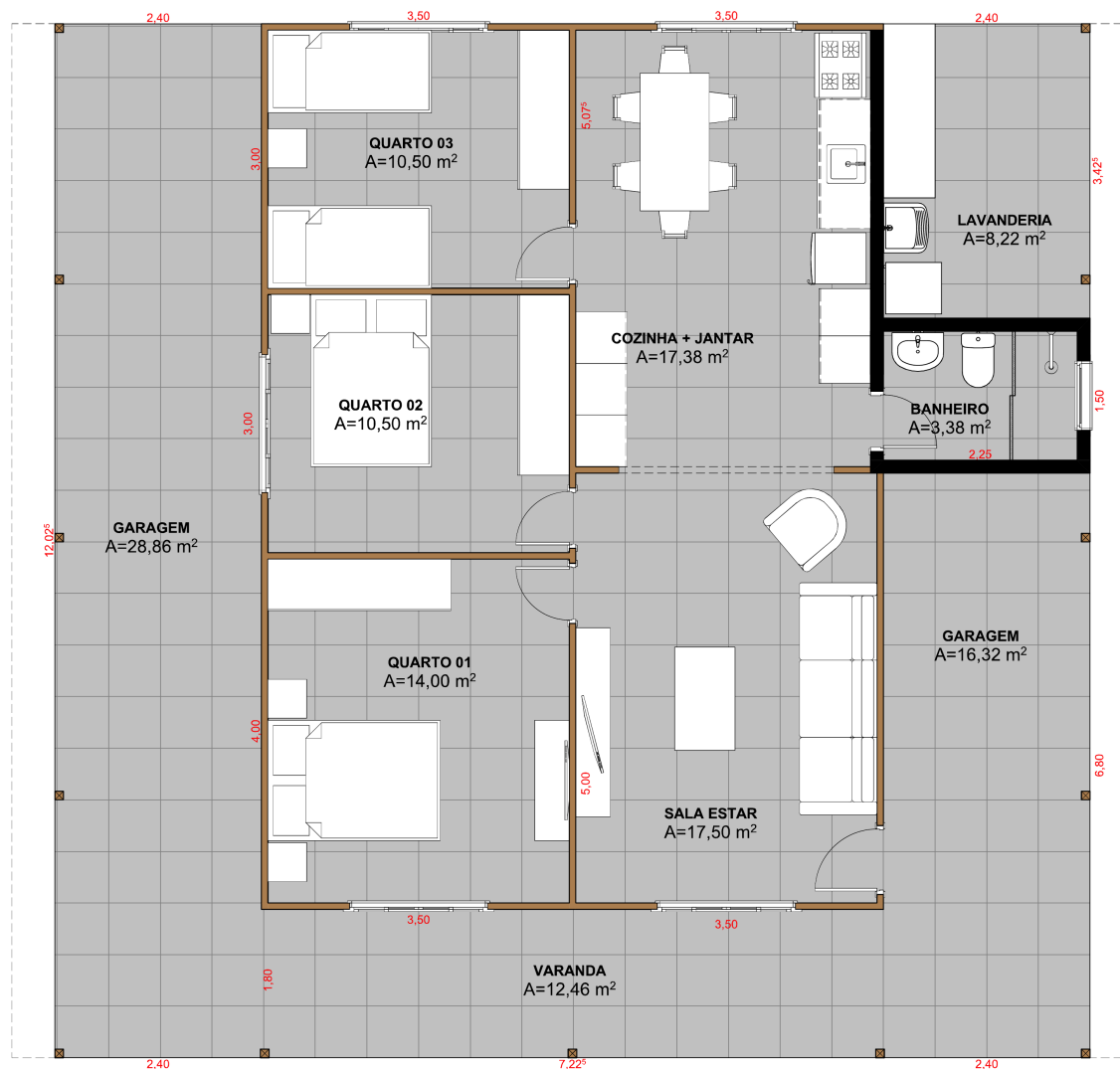
Modelo 79 • Casa Modelo Chácara Praia (7x10 tipo 02) • Marca atualizada para Construtora Silva.
