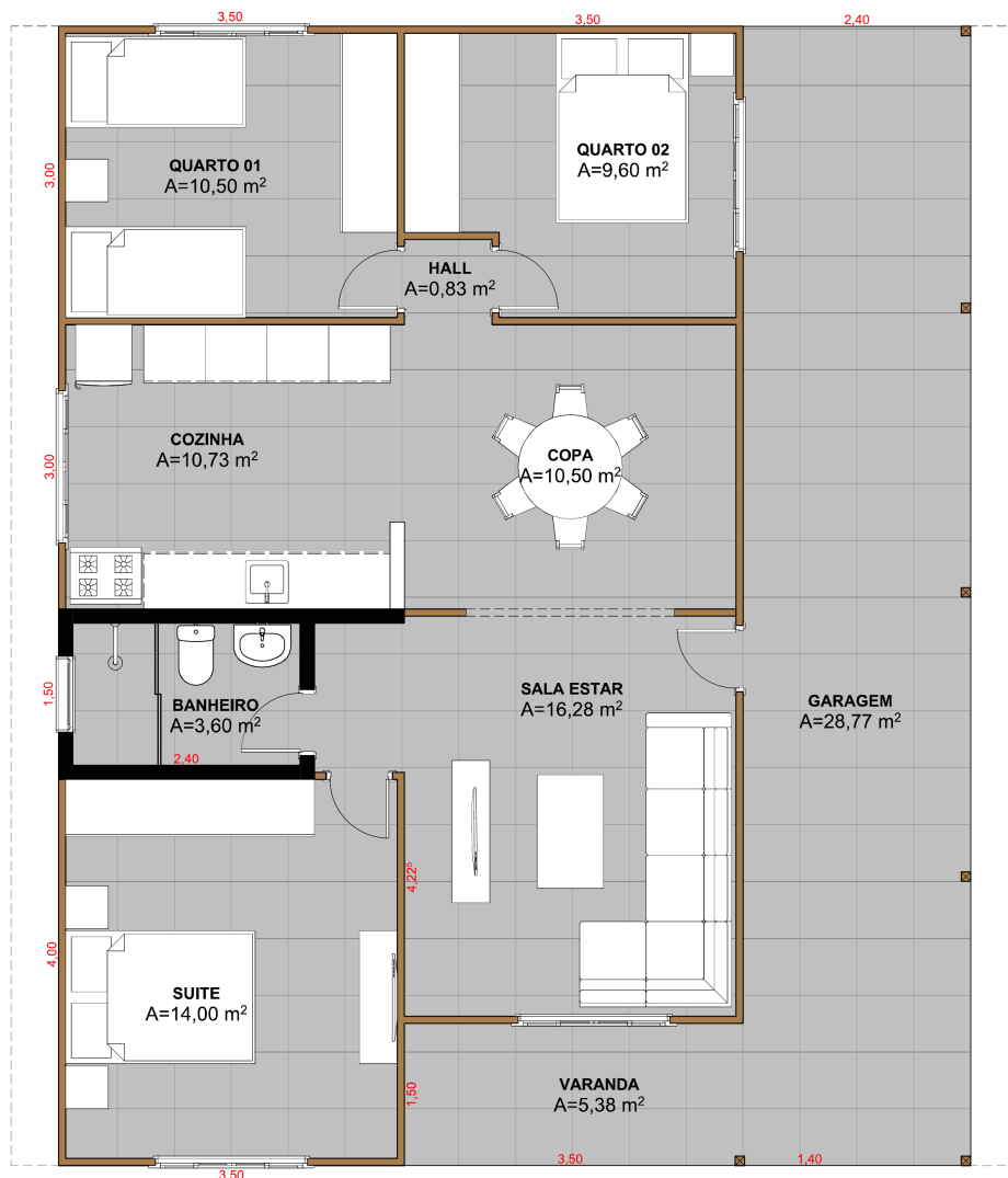
Modelo 44 • Casa Modelo Família (7x10) • Marca atualizada para Construtora Silva.
