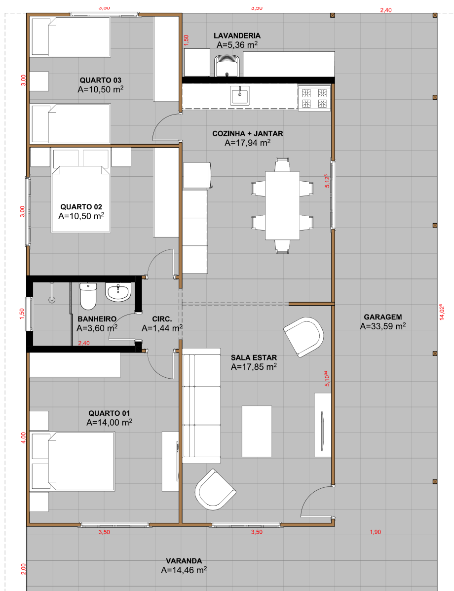
Modelo 16 • Casa Modelo Frente Dupla (7x10) • Marca atualizada para Construtora Silva.
